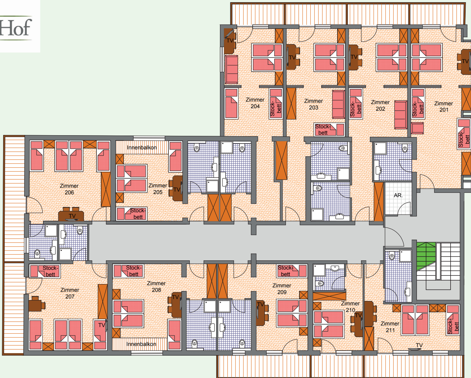
HAUPTHAUS-SÜDSEITE 2. Stock
